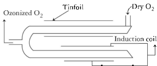
Fig. 6.1 Siemens's Ozonizer
