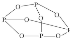
Fig. 5.16 St. of P_4O_6
