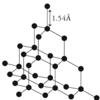
Fig. 3.7 Diamond
